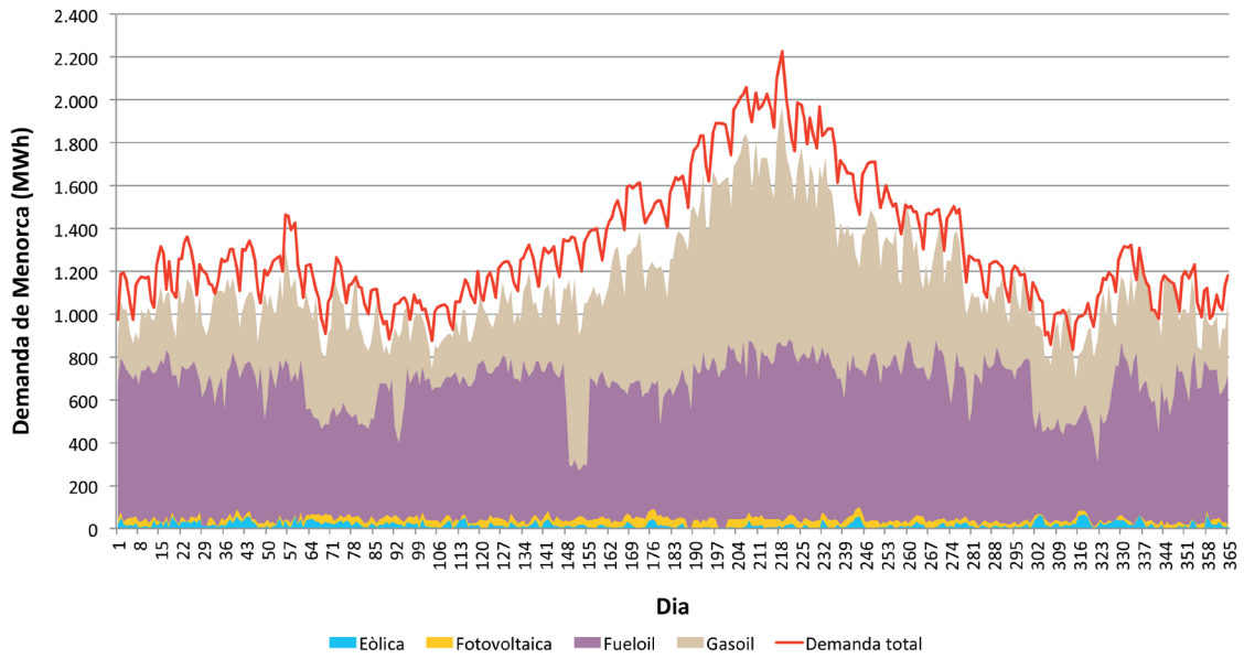
▲ Figura 5.3. Cobertura de demanda elèctrica diària de l'any 2013. La diferència entre la corba de demanda total i la producció acumulada de sota correspon als intercanvis Mallorca-Menorca via cable submarí. Font: Elaboració pròpia a partir de dades de Red Eléctrica de España.
