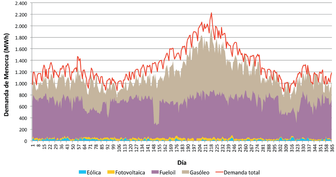
▲ Figura 5.3. Cobertura de demanda eléctrica diaria del año 2013. La diferencia entre la curva de demanda total (línea roja) y la producción acumulada de debajo corresponde a los intercambios Mallorca-Menorca vía cable submarino. Fuente: Elaboración propia a partir de datos de Red Eléctrica de España.
