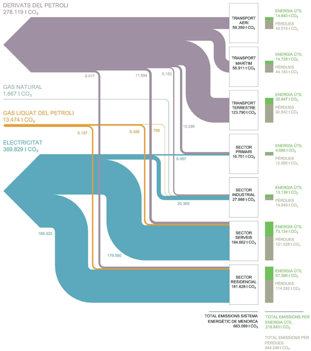
▲ Figura 8.3. Diagrama de Sankey d'emissions directes de CO 2 del sistema energètic de Menorca de l'any 2013, per sectors. Unitats: tones de CO 2 (t CO 2 ). Font: Elaboració pròpia.
