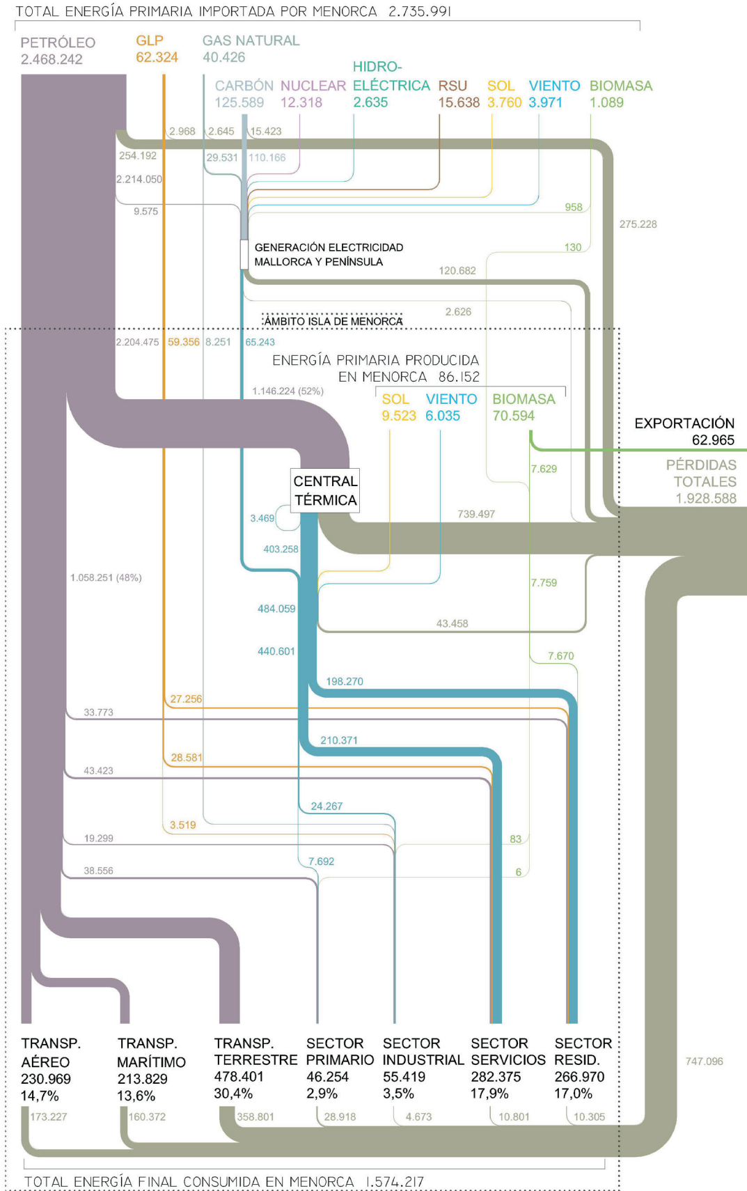
▲ Figura 4.1. Diagrama de Sankey del sistema energético de Menorca, año 2013. Fuente: Elaboración propia.
